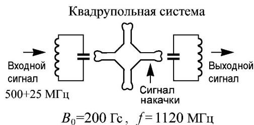
Рис. 3. Схема резонансной лампы Адлера
