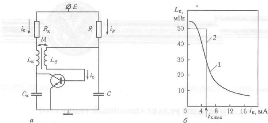
Рис. 1, а. Схема генератора: L_k = 50 мГн, L_b = 0.5 мГн, C_k = 3600 пФ, C = 0.047 мкФ, E = 7 В
