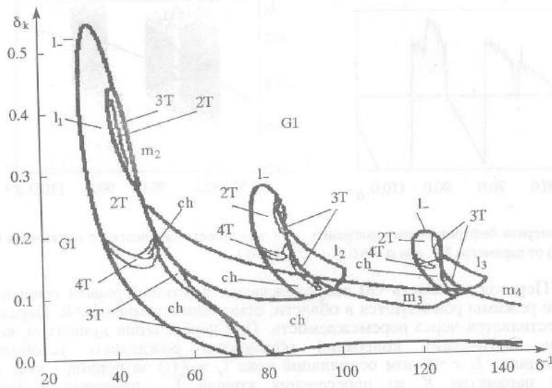
Рис. 3. Бифуркационная диаграмма отображения (12)
