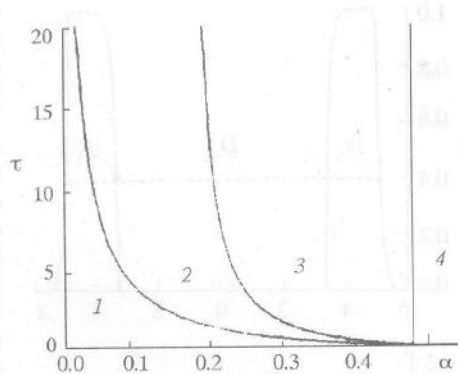
Рис. 10. Области существования локализованных структур на плоскости параметров нейроподобной среды для U_p=0.5 . В области 1 существуют только неподвижные локализованные структуры и один тип фронта переключения. В областях 2,3,4 при \tau \geq 1 существуют бегущие импульсы и три типа фронта переключения. В области 3 при \tau \leq 10 существуют локализованные пульсирующие структуры. В области 4 все неподвижные структуры подавлены воздействием локального порога возбуждения
