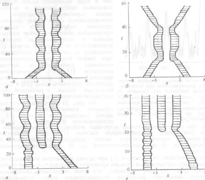
Рис. 11. Некоторые сценарии образования (а,б), распада (в) и подавления (з) пульсирующих очагов в результате столкновения бегущих импульсов
