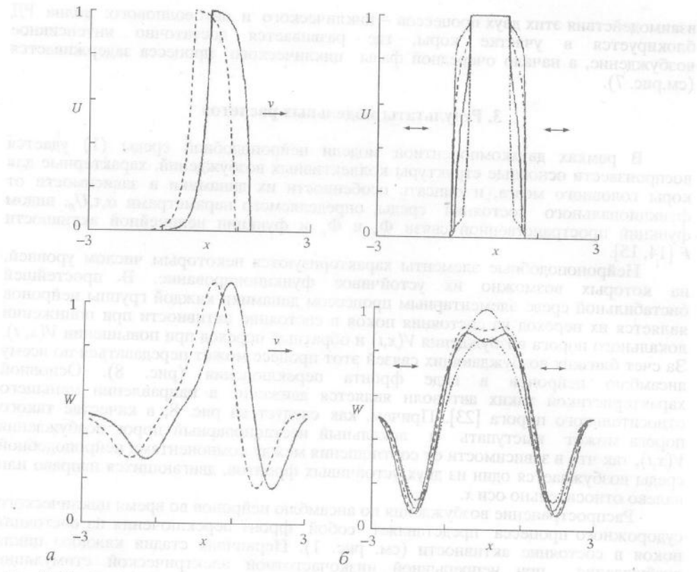
Рис. 9. Профиль локализованных динамических структур для локальной U(x,t) и усредненной W(x,t) = \int_{-\infty}^{+\infty} dx' \Phi_u(x'-x)U(x',t) - \alpha V(x,t) переменных активности нейроноподобных элементов: а - бегущий импульс; б - пульсирующая автоструктура
