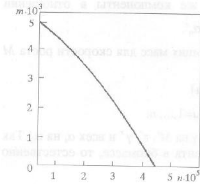
Рис. 4. Кривая производственных возможностей. По оси ординат отложено количество роботов m , по оси абсцисс – количество штук пиццы n
