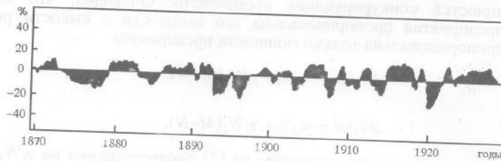
Рис. 2. Цикличность развития американской экономики. По оси ординат отложены в процентах отклонения от линии, обозначающей долгосрочную тенденцию экономической активности
