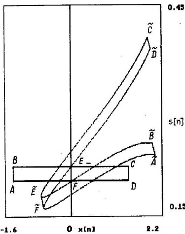
Рис.7. Преобразование отображением (7) узкого прямоугольника ABCD = \{x \in [-1.4; 1.4], s \in [0.2; 0.22]\} в криволинейный прямоугольник A'B'C'D' ( \omega_0^2 = 0.56 , \gamma = 0.85 , H = 0.0 , p = 4.0 )
