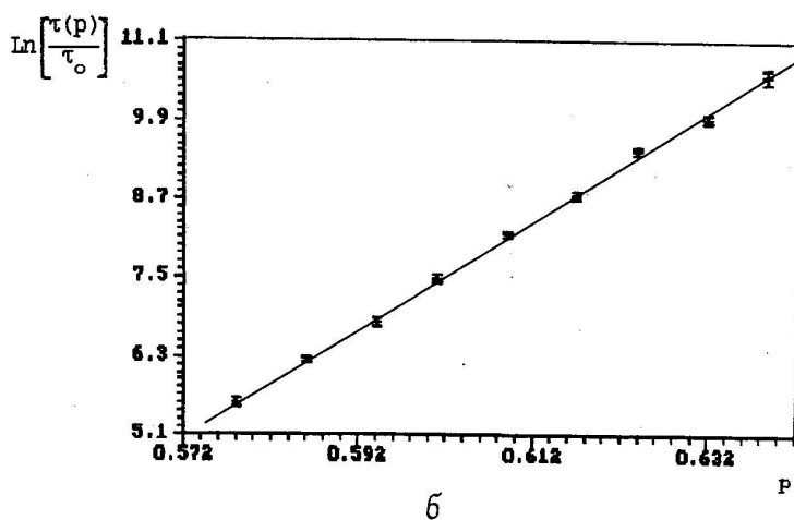
Рис.4. Экспериментальные зависимости \ln[\frac{\tau(p)}{\tau_0}] ( \tau_0=1\text{мс} ) от p : а - для НЧ-макета (8 звеньев), б - для ВЧ-макета (9 звеньев)
