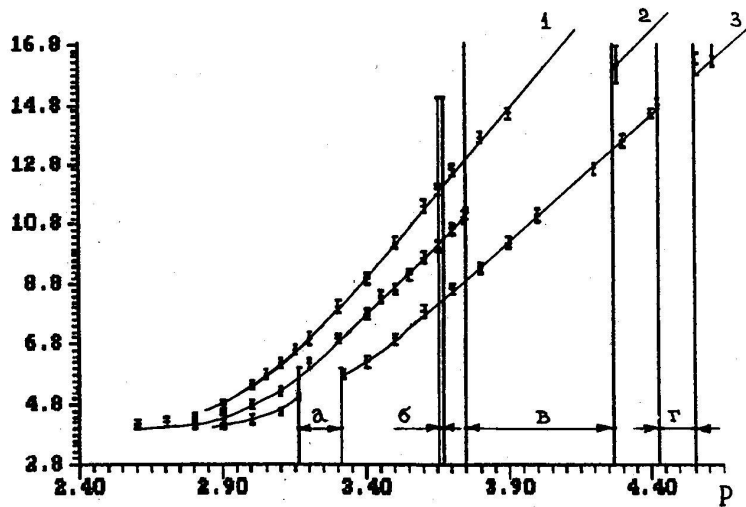
Рис.6. Зависимости \text{Ln}[\langle n \rangle] для ПХ в отображении (7) при различных величинах асимметрии нелинейности (6): 1 - \alpha = -0.1 , 2 - \alpha = 0.0 , 3 - \alpha = 0.1 ; вертикальными полосами показаны окна периодичности: а - \Delta_1 ( \alpha = 0.1 ), б - \Delta_2 ( \alpha = -0.1 ), в - \Delta_3 ( \alpha = 0.0 ), г - \Delta_4 ( \alpha = 0.1 )
