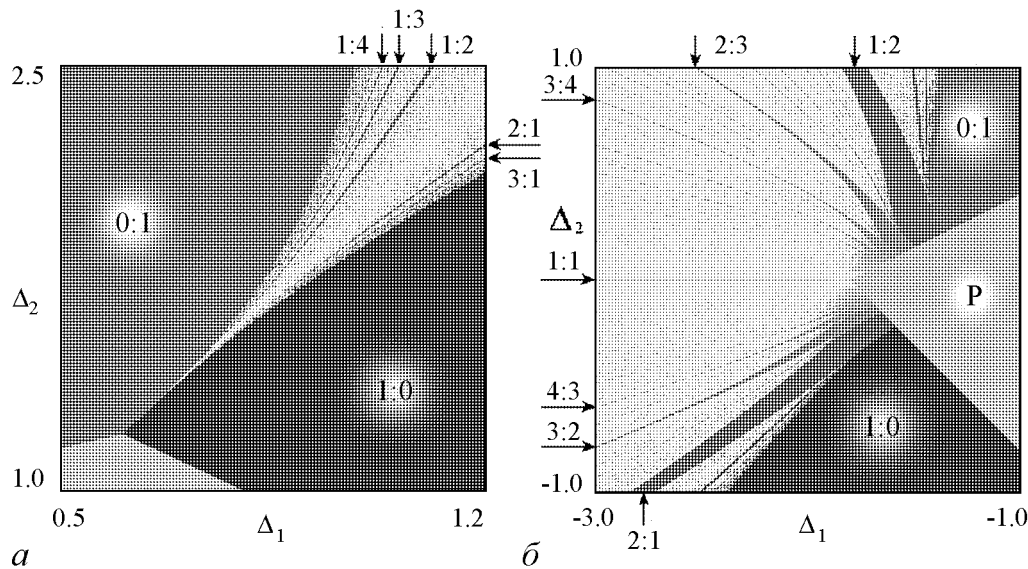
Рис. 4. «Карты торов» в окрестности точек SNF (а) и ASNF (б). В виде дробей показаны числа вращения, характеризующие инвариантные кривые
