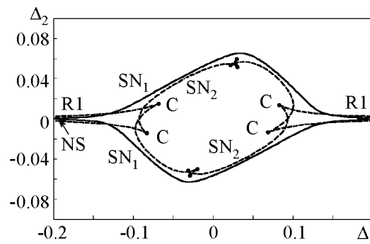
Рис. 5. Бифуркационные линии системы трех связанных осцилляторов ван дер Поля (1), \lambda = 0.1 , \mu = 0.04 . SN_1 – седло-узловая бифуркация устойчивого предельного цикла, SN_2 – неустойчивого, C – точка сборки, NS – линия Неймарка-Сакера, R1 – резонанс 1:1
