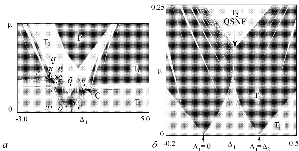
Рис. 10. a – карта ляпуновских показателей четырех фазовых осцилляторов (10); б – ее увеличенный фрагмент; \Delta_2 = 0.3 , \Delta_3 = 1
