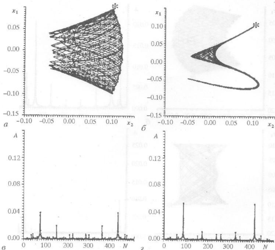
Рис. 10. Траектории на координатной плоскости (x_1, x_2) (а, б) и соответствующие им спектры в отн. ед. (z, z) при наличии потенциала Леннарда - Джонса (3) с параметрами (в отн. ед.): \rho = 1 , \sigma = 0.05\sqrt{10} , (x_1^L, x_2^L) = (0, -0.2) ; а, в - все пружины линейны (квадратичные потенциалы) и одинаковы; б, z - квадратичные потенциалы были заменены на потенциалы Морзе при соответствии параметров
