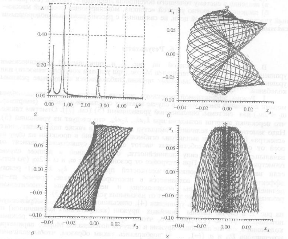
Рис. 4. График зависимости амплитуды A огибающей (отн.ед.) от коэффициента кратности собственных частот h = \omega_1/\omega_2 , возведенного в квадрат при начальных условиях для каждой точки графика (x_1, dx_1/dt, x_2, dx_2/dt) = (-0.1, 0, 0, 0) отн.ед. (а) и траектории системы на координатной плоскости (x_1, x_2) для каждого из трех резонансных состояний (б, в, г). Координаты начальных условий на плоскости (x_1, x_2) помечены звездочкой. Графики строились для случая уравнений (4) (потенциалы Морзе)
