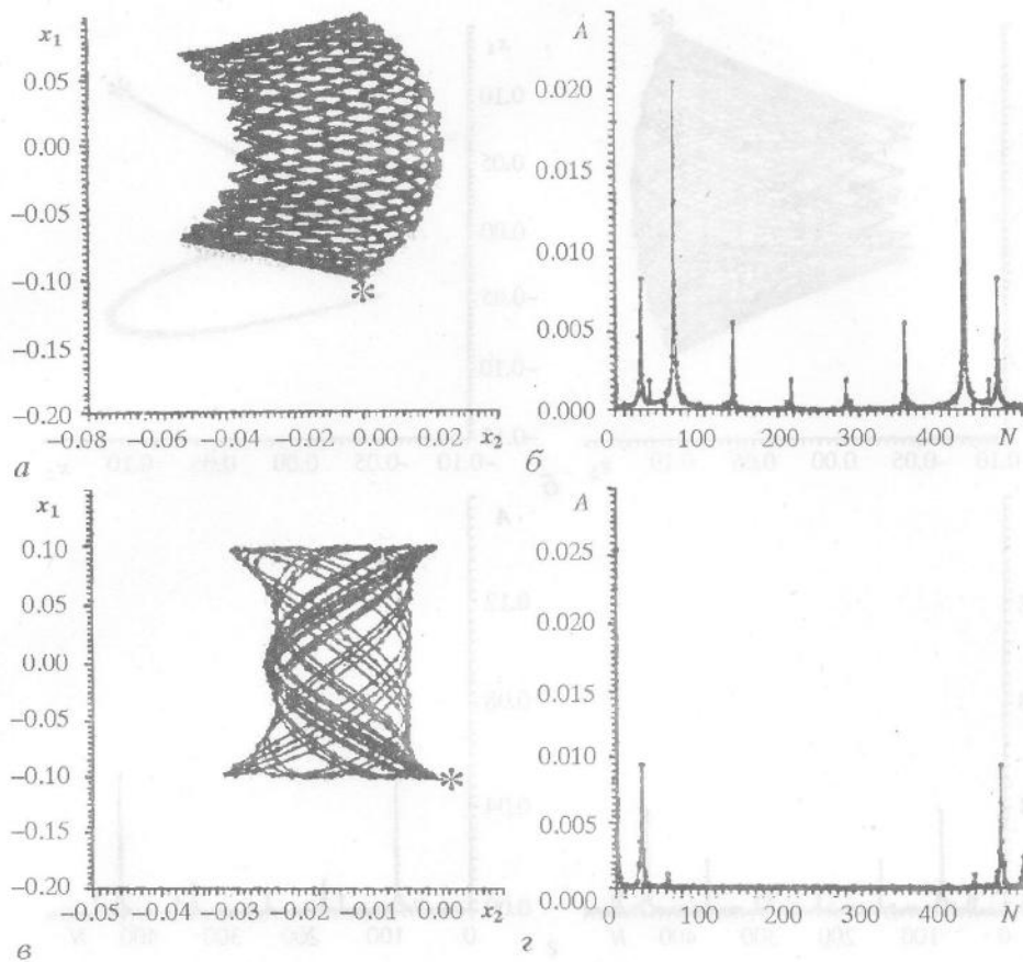
Рис. 9. Траектории системы на координатной плоскости (x_1, x_2) и соответствующие спектры при наличии потенциала Леннарда – Джонса (3) с параметрами (в отн.ед.): a, б - \rho=0.01, \sigma = 0.05\sqrt{10}, (x_1^L, x_2^L) = (0, -0.2) ; в, г - \rho = 0.015, \sigma = 0.05\sqrt{10}, (x_1^L, x_2^L) = (0, -0.2) . Координаты начальных условий на плоскости (x_1, x_2) помечены звездочкой, пружины линейны и выполняется условие резонанса
