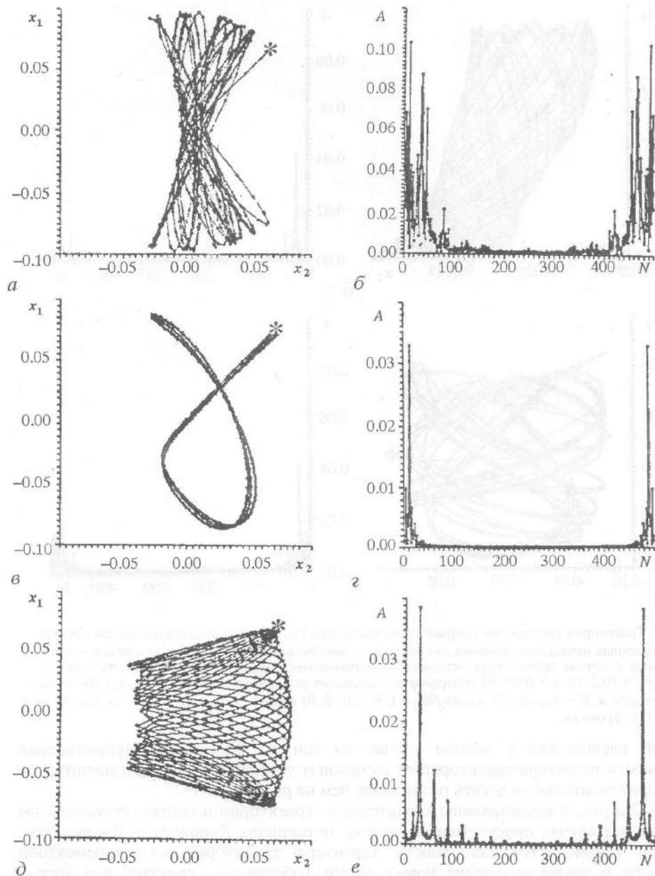
Рис. 7. Траектории системы на координатной плоскости (x_1, x_2) и соответствующие им спектры для случаев: а, б – в систему (рис. 2, а) вместо потенциала (3) введена абсолютно упругая выпуклая «стенка» с координатами центра и радиусом соответственно: (x_1^L, x_2^L) = (0, -0.2) , r = 0.05\sqrt{15} ; в-е – в системе присутствует потенциал Леннарда – Джонса с параметрами: \rho = 0.001 , \sigma = 0.05\sqrt{15} , (x_1^L, x_2^L) = (0, -0.2) (в, г); \rho = 10 , \sigma = 0.05\sqrt{10} , (x_1^L, x_2^L) = (0, -0.2) (д, е). Во всех случаях а-е пружины линейны и одинаковы. Координаты начальных условий на плоскости (x_1, x_2) помечены звездочкой
