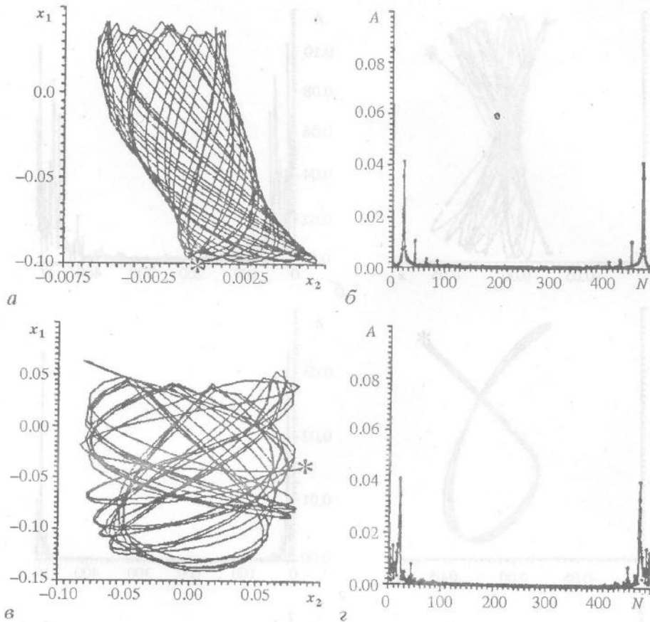
Рис. 8. Траектории системы на координатной плоскости (x_1, x_2) и соответствующие им спектры при различных начальных условиях для системы с линейными пружинами и выполнении условия резонанса в случае присутствия «стенки» с координатами центра и радиусом соответственно: (x_1^L, x_2^L) = (0.2, 0) , r = 0.05\sqrt{10} (координаты начальных условий на плоскости (x_1, x_2) помечены звездочкой); а, б - (x_1, \partial x_1/\partial t, x_2, \partial x_2/\partial t) = (-0.1, 0, 0, 0) отн.ед.; в, з - (x_1, \partial x_1/\partial t, x_2, \partial x_2/\partial t) = (0, 0, 0.1, 0) отн.ед.
