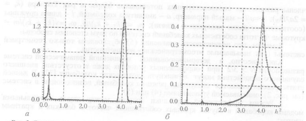
Рис. 3. Зависимость амплитуды A огибающей (отн.ед.) от коэффициента кратности собственных частот h = \omega_1/\omega_2 , возведенного в квадрат. Максимумы соответствуют режимам наиболее эффективной перекачки энергии при \omega_1 = \omega_2/2 и \omega_1 = 2\omega_2 . График строился для случая уравнений (5) (квадратичные потенциалы). Начальные условия в каждой точке графика: (x_1, dx_1/dt, x_2, dx_2/dt) = (-0.1, 0, 0, 0) отн.ед. (а); (x_1, dx_1/dt, x_2, dx_2/dt) = (0, 0, -0.1, 0) отн.ед. (б)
